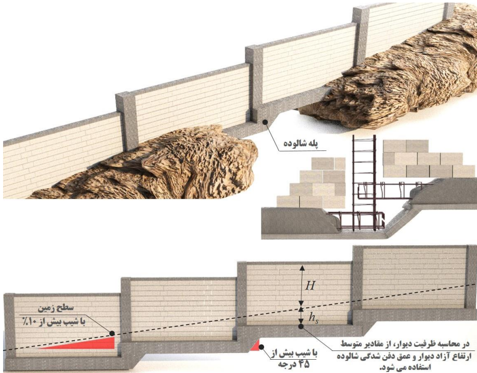
شکل ۵-۳ نحوه اجرای پله‌های دیوار محوطه در زمین با شیب بیش از ۱۰٪
