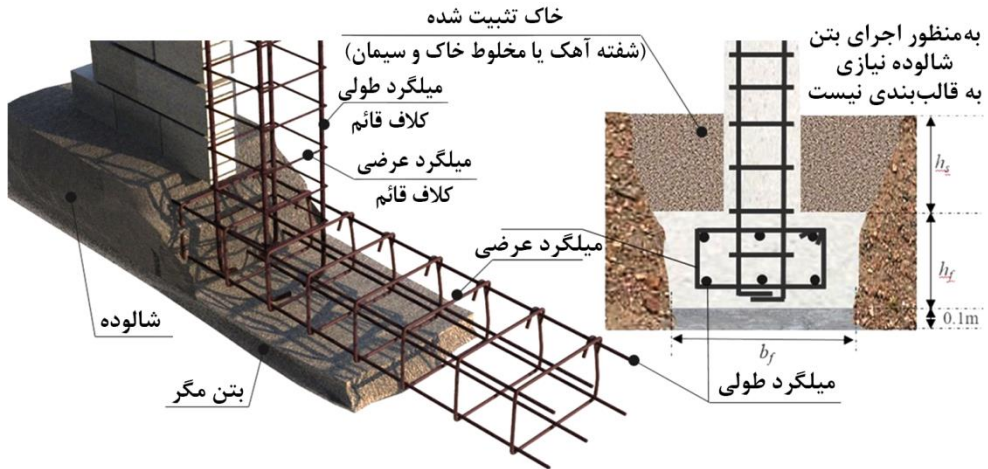
شکل ۴-۷ جزئیات اجرا و آرماتوربندی شالوده
