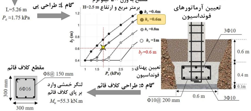
شکل ۴-۹ روند گام به گام طراحی دیوار محوطه بر اساس دستورالعمل
