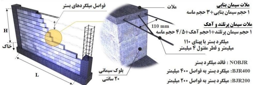
شکل ۴-۲ ظرفیت خارج از صفحه پانل بنایی ۲۰ سانتی ساخته شده از بلوک‌های سیمانی توخالی
